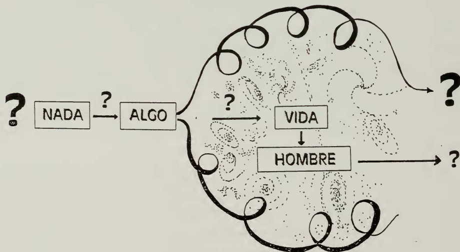
Figura 1. Representación esquemática del proceso global del origen del Universo y del hombre. (Explicación y comentarios, en el texto).
